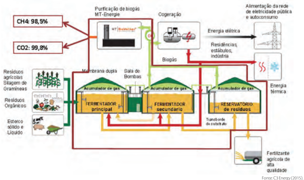
FIGURA 14 | Esquema de funcionamento do Biodigestor Alemão em duas etapas.
