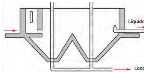
FIGURA 03 | Equalizador/Decantador
